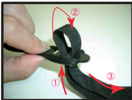
⑩カバー前後にあるベルトは図の①から③の順に通し、③で通したベルトを引っ張る事で締まります。カバーの前後を締め込み固定します。
