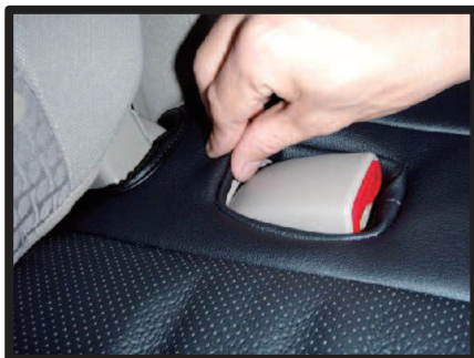
⑤シートベルトの受け部分の生地は中に入れ込みます。
