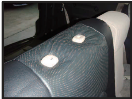
④ヘッドレストの台座部分を穴から取り出します。
