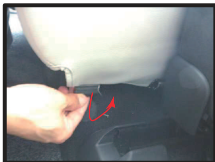
⑰カバー内側面に付いているプラスチックフックを7ページの⑭を参考にシート裏で固定します。
