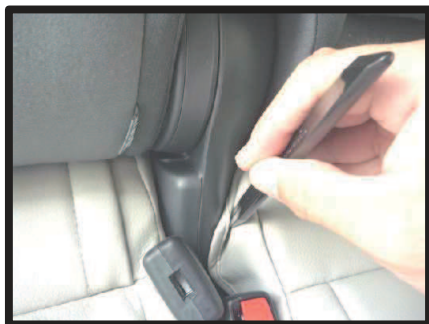
⑯シートの付け根部分の生地を、ヘラなどを使用してシートとプラスチック部の隙間に入れ込みます。
