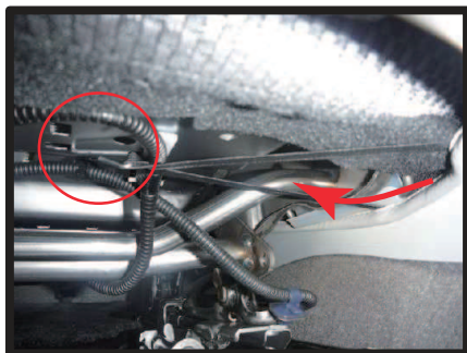
⑦ S字フックを取り付けたゴムを座面下に引っ掛け固定します。
