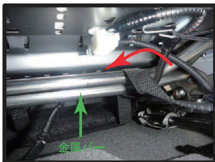
⑧ カバー前側に付いているベルトを、座面下を通し、後ろ側へ引き出します。この際、図のように金属バーの上側を通すようにします。
