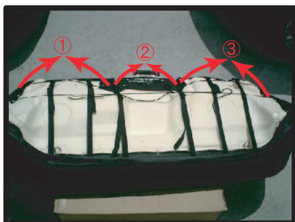
⑫ゴムは写真の①②③の3箇所、①の方法で固定します。
